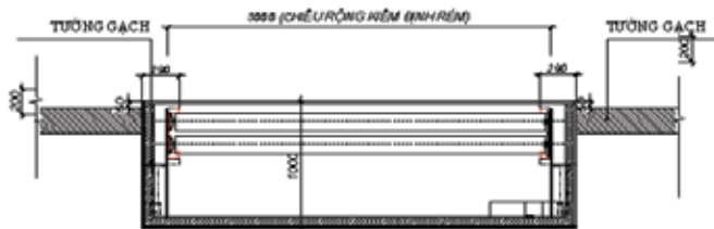
MẶT CẮT 1-1
