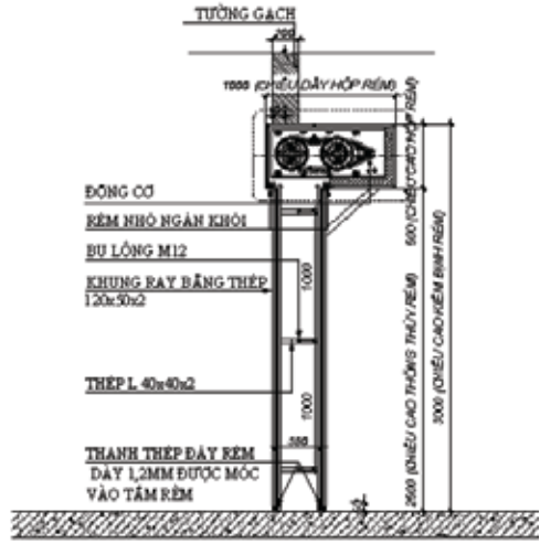
MẶT CẮT 3-3
